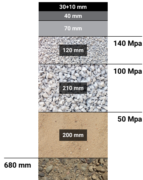
1. Traditsiooniline maantee
