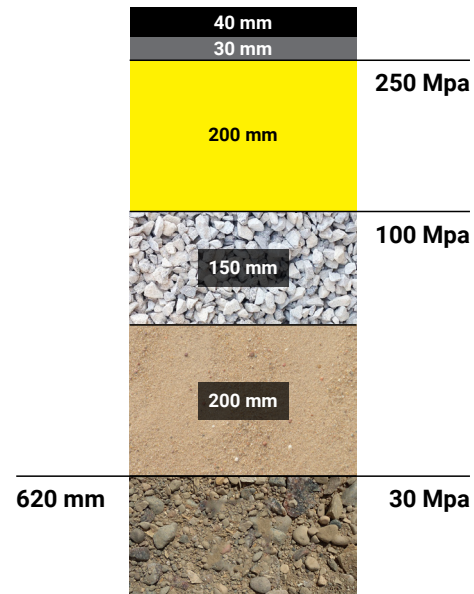
2. StabilRoad® maantee
