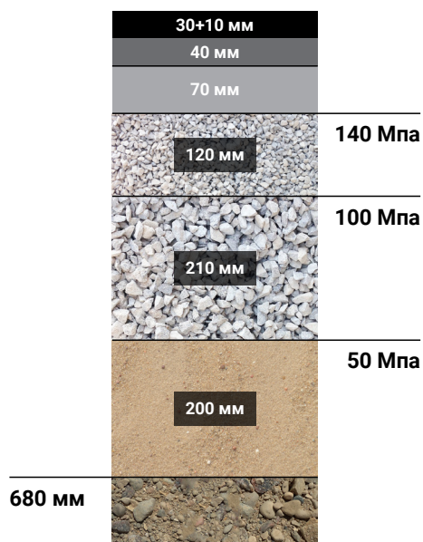
1. Традиционная дорога
