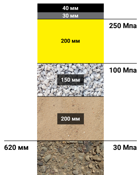
2. StabilRoad® дорога
